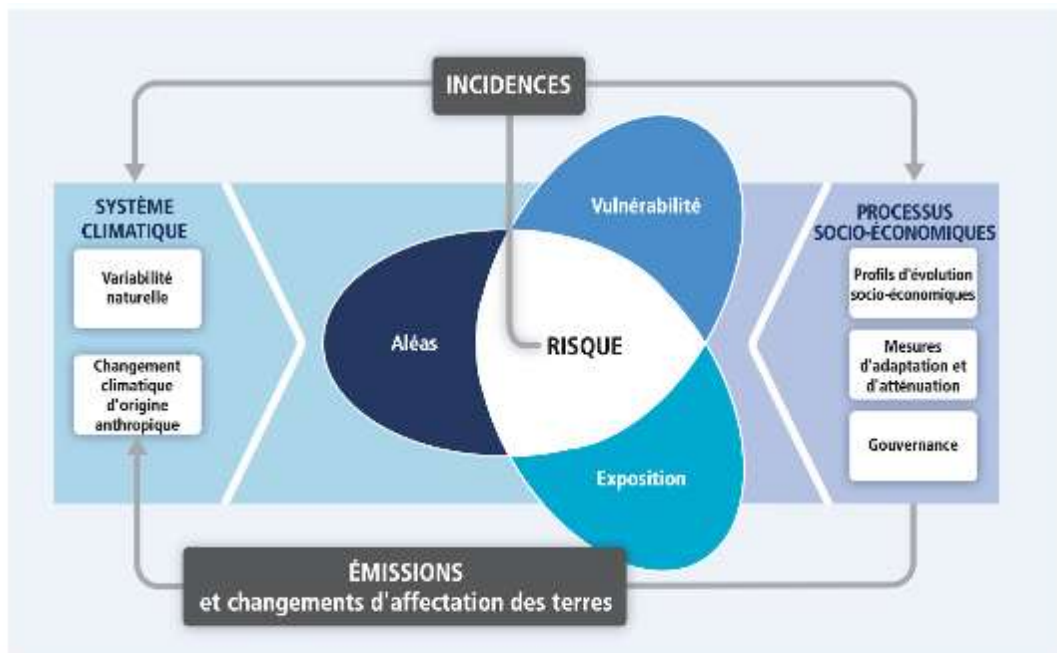
Figure RID.1 | Notions essentielles abordées dans la contribution du Groupe de travail II au cinquième Rapport d'évaluation (GTR RES). Le risque d'incidences liées au climat découle de l'interaction entre des aléas climatiques (y compris les tendances et les phénomènes dangereux) et la vulnérabilité et l'exposition des systèmes anthropiques et naturels. Les changements qui touchent à la fois le système climatique (à gauche) et les processus socio-économiques, y compris l'adaptation et l'atténuation (à droite), sont les principaux causes des aléas, de l'exposition et de la vulnérabilité. (19.2, figure 19-1)
