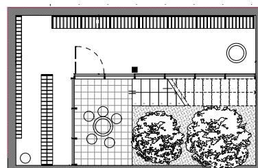
Plan du sous-sol © Anaïs Magnabal architecte
