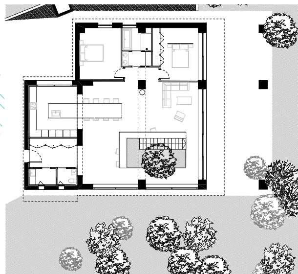
Plan du rez-de-jardin © Anaïs Magnabal architecte
