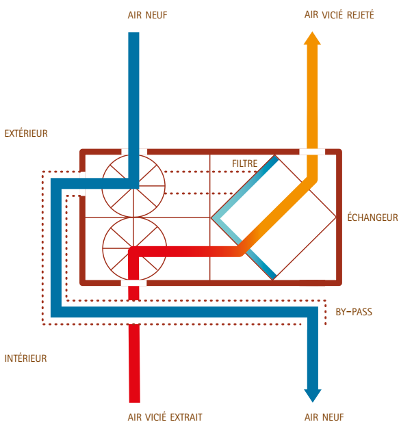
> FONCTIONNEMENT D'UN CAISSON VMC DOUBLE FLUX ÉQUIPÉ D'UN BY-PASS EN POSITION ÉTÉ
