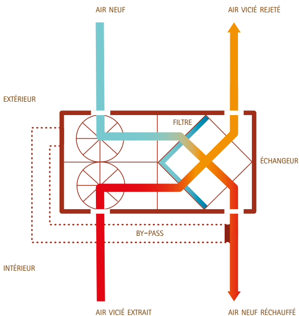
> FONCTIONNEMENT D'UN CAISSON VMC DOUBLE FLUX ÉQUIPÉ D'UN BY-PASS EN POSITION HIVER
