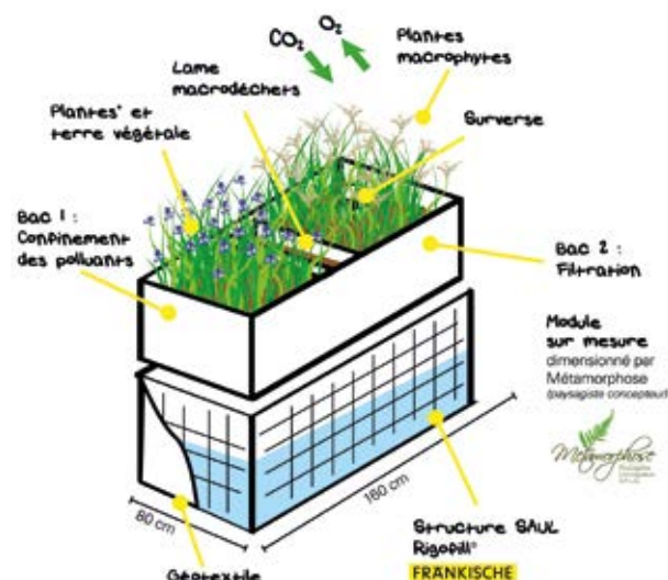
Schéma de principe des trois bacs
